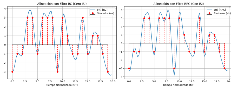
Figura 7: Alineación de los Filtros RC y RRC .
