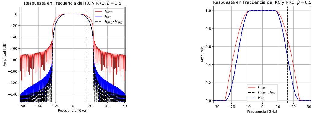
Figura 6: Respuesta en frecuencia de un RRC y un RC . \beta = 0,5 .
